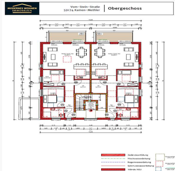
Grundriss OG
